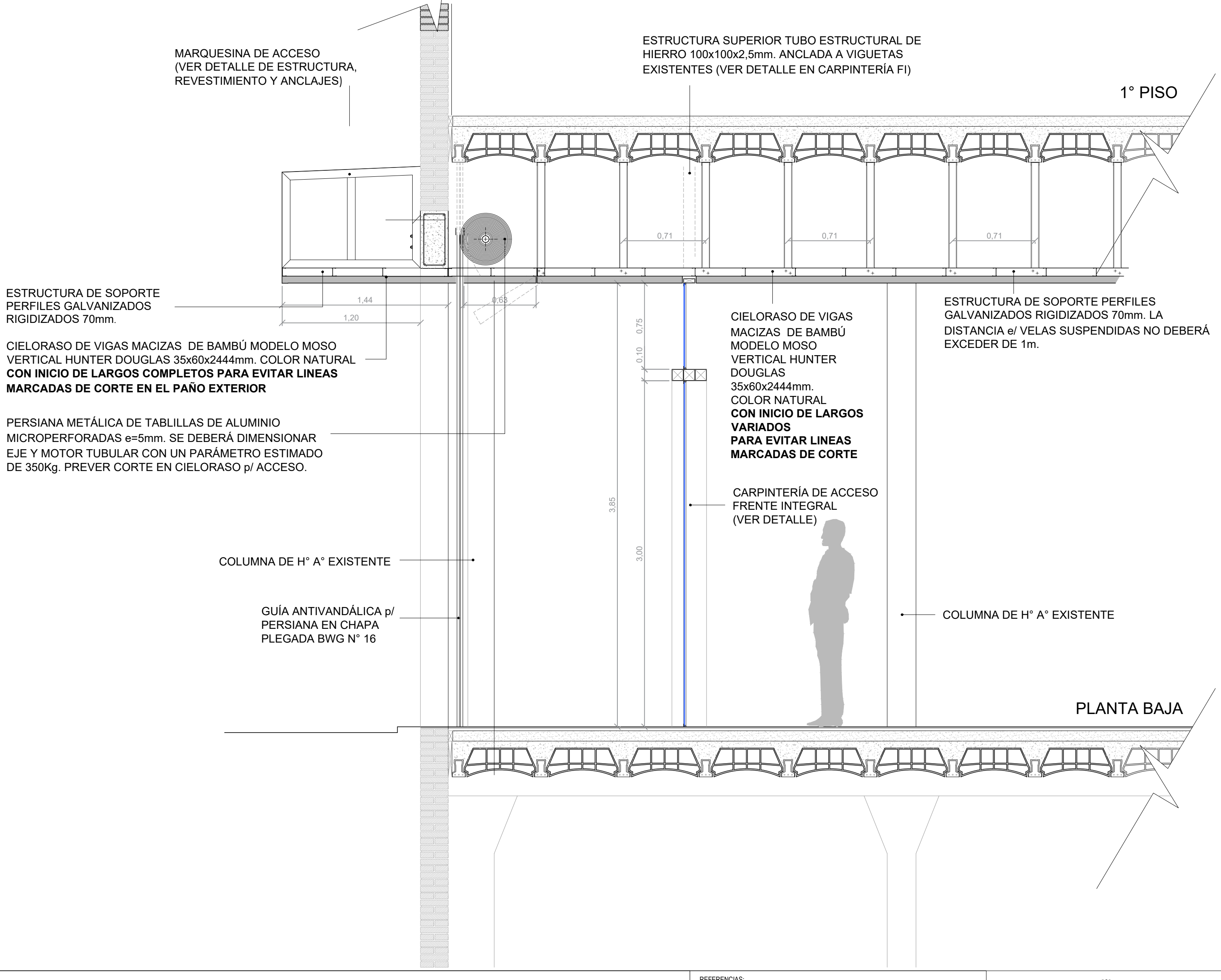
CORTE A-A
