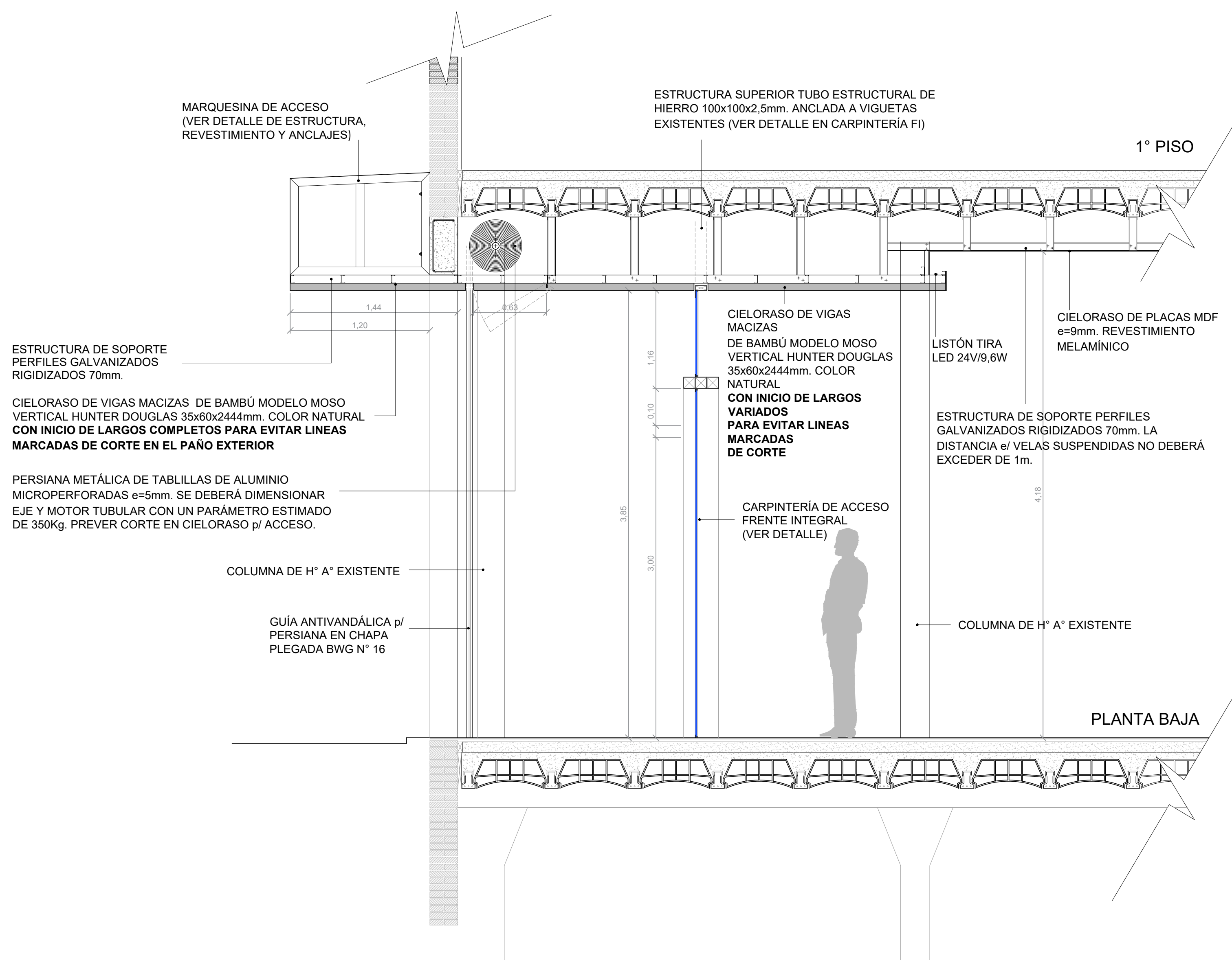
CORTE B-B
