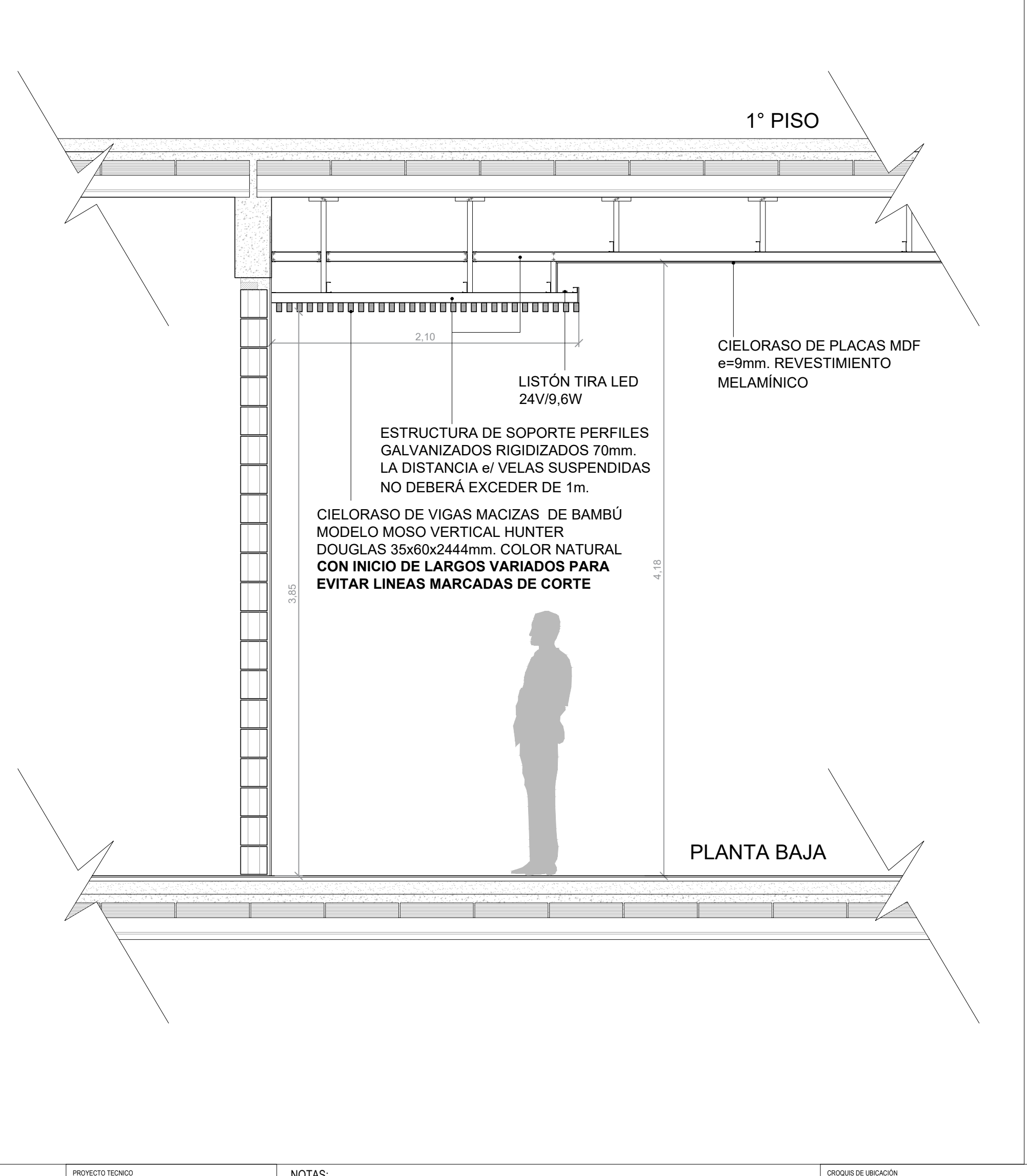
CORTE C-C
