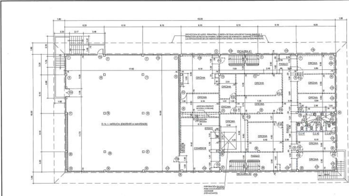
PLANTA ARQUITECTONICA EXISTENTE / DEMOLICION - PRIMER ALTO - (NIVEL 100) - EL BOSTOS VERTICALES FUE UN AQUEL INDICADO EN LA OFICINA.
